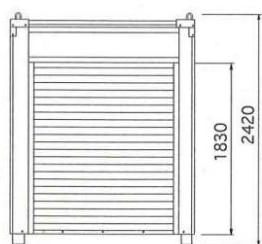
トランクルーム寸法図・14基
